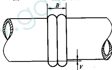
图 5.2.4-1 翻边对称性示意
